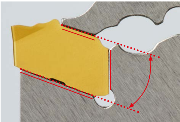
Konuswinkel
